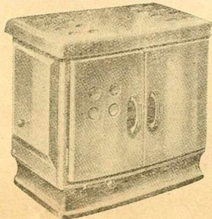
104. SAINT-NICOLAS. MIDINETTE. Deux appareils en un seul à feu continu, permettant la cuisine et le chauffage; émail bleu, castor ou brun, avec ou sans charbonnier. L : 60 cm.
