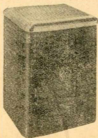
109. SAINT-JEAN. Poêle à mazout à thermostat breveté, faible consommation. Chauffe 40 à 150 m 2
