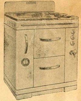
4. DEVILLE. Cuisinière mixte, charbon, bois, gaz, entiè- rement fonte, 2 fours, un à charbon, un à gaz. L : 72 cm.
