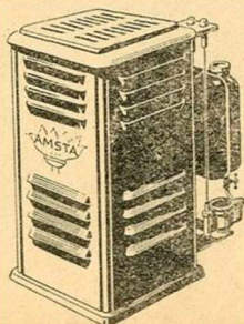
110. AMSTA modèle 84. Poêle à mazout à tirage naturel, tôle émaillée. Chauffe 120 m 2 .
